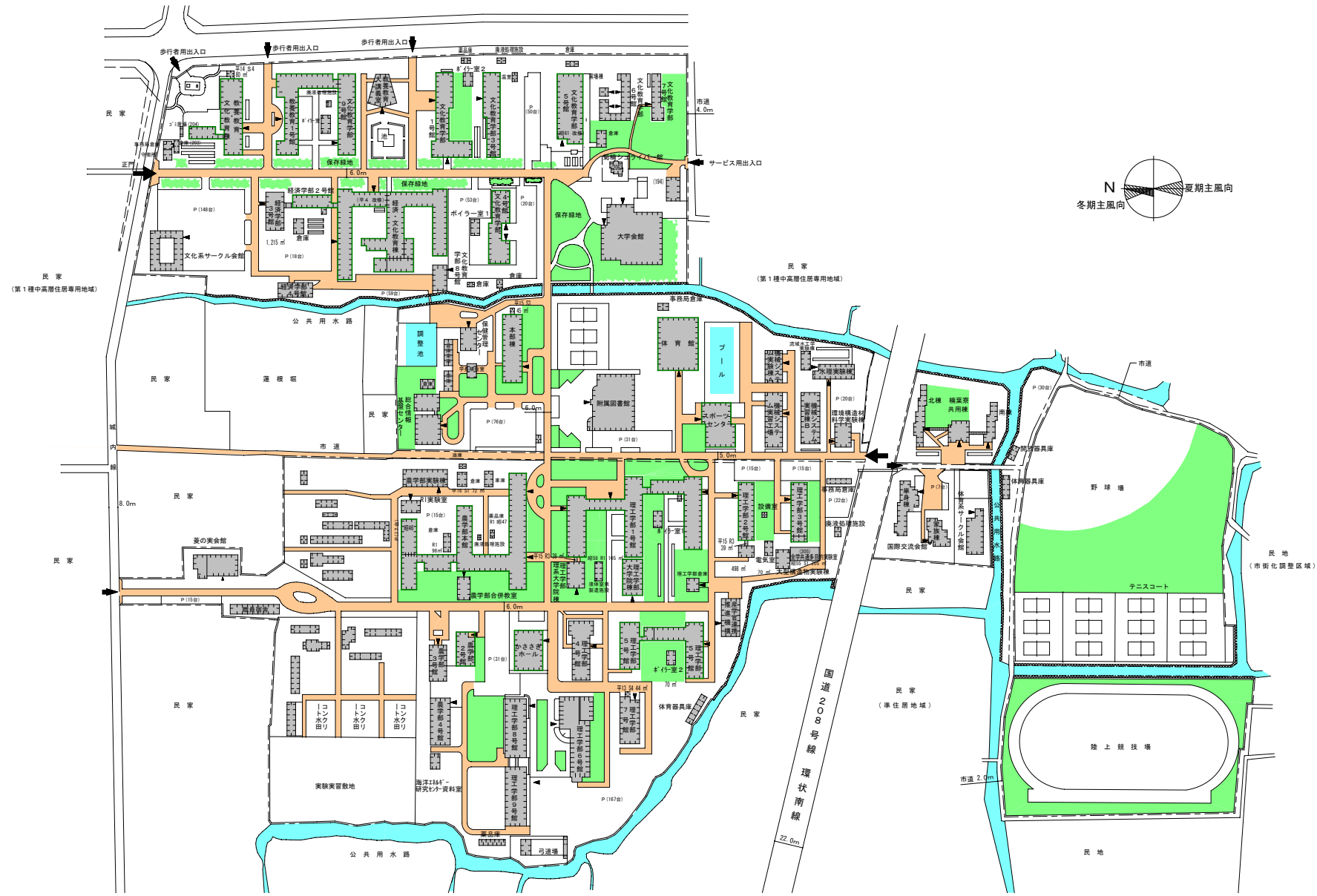
配置図 S=1/3,000
